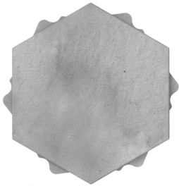
ASAK FLYT 10 286x312x80 mm Units per m 2 : 12,84 Weight per m 2 : 158,6kg
